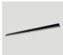
规格: 1200泛光灯 功率: 48W 色温: 白光/中性光/暖光/变光 尺寸: 1207*22*25mm
